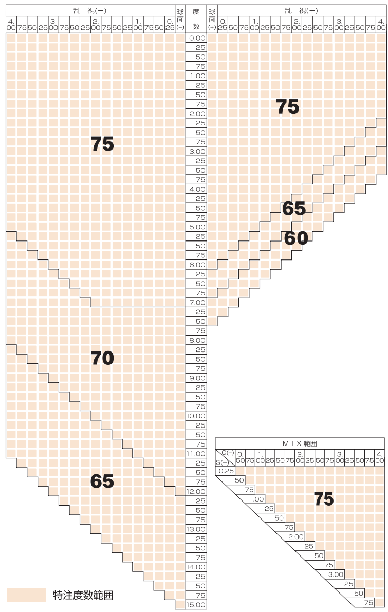
累進帯長 9mm レンズタイプ スタンダード のレイアウト図
