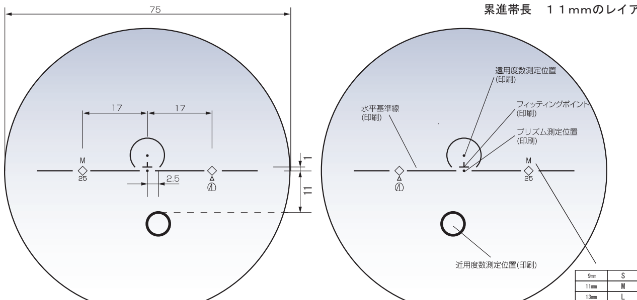
累進帯長 1.1 mmのレイアウト図
