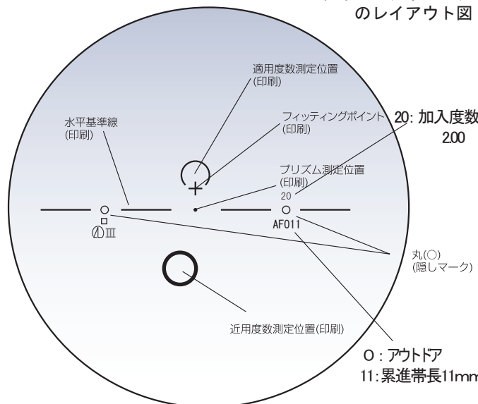
外径75mm、UV3G生材、累進帯長 11mm レンズタイプ アウトドア のレイアウト図
